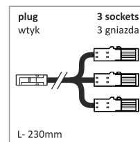
LED cable with MINI 3 sockets and 1 plug / black rozdzielacz LED MINI 3xG/1xW / czarny 2x0,35; L-230
