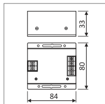
LED 2 channel warm-cold receiver moduł sterujący LED ciepły-zimny 2 kanałowy 12V/24VDC; 144W/288W
