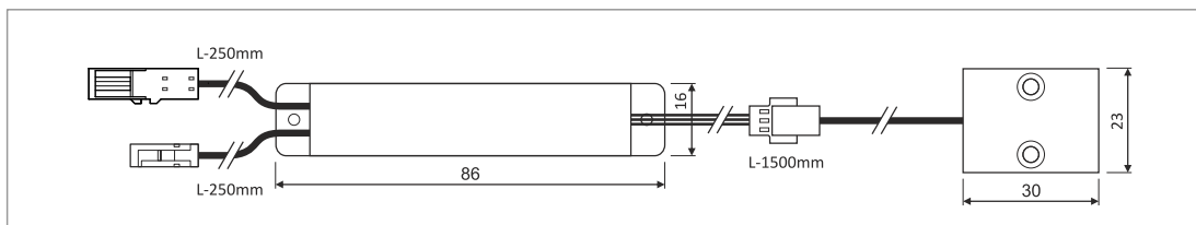
door operated sensor switch włącznik bezdotykowy drzwiowy 12-24V/30W
