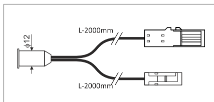
touch sensor ON/OFF switch włącznik dotykowy ON/OFF 12V/30W
