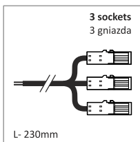
LED cable with 3 MINI sockets / black rozdzielacz LED MINI 3xG / czarny 2x0,35; L-230
