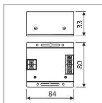
LED 3 channel RGB receiver moduł sterujący LED RGB 3 kanałowy 12V/24VDC; 216W/432W
