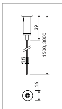
SKB sling zawiesie SKB
