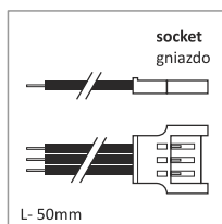
LED cable with socket przewód LED 1xG 3x0,22; L-50; MIKRO3; 1xG
