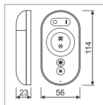
LED RGB remote controller pilot sterujący LED RGB
