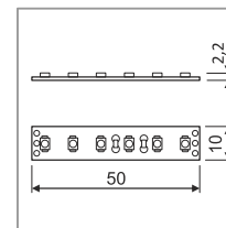
LED strip 3528 warm-cool white (B) taśma LED 3528 biały ciepły-zimny (B) 12V; 9,6W/m; 120P/m
