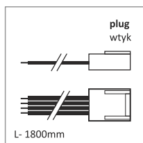
LED RGB cable with plug przewód LED RGB 1xW 4x0,5; L-1800; MIKRO4
