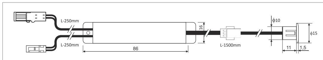
hand operated sensor switch włącznik bezdotykowy ręczny 12-24V/30W
