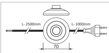
cable with footswitch and plug / black przewód z włącznikiem nożnym / czarny 250V; 2x0,75; 2,5A; L-1000/2500
