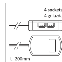
LED RGB 4 way distribution box rozdzielacz LED zintegrowany RGB 4xG 4x0,5; L-200; MIKRO4
