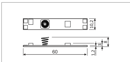
touch LED INSIDE dimmable switch włącznik dotykowy ściemniający LED INSIDE 12-24V/36W
