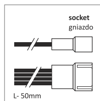
LED RGB cable with socket przewód LED RGB 1xG 4x0,5; L-50; MIKRO4
