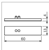
LED SU/GR/CO dimmable, touchless switch włącznik LED SU/GR/CO ściemniający bezdotykowy 12-24V/35W
